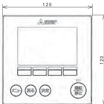
外形図
